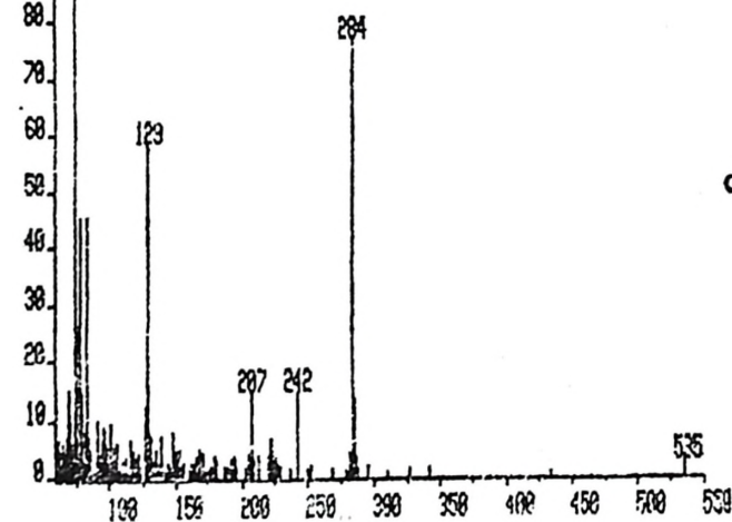
Slika 4. Spektogram masa hromatografskog signala C
